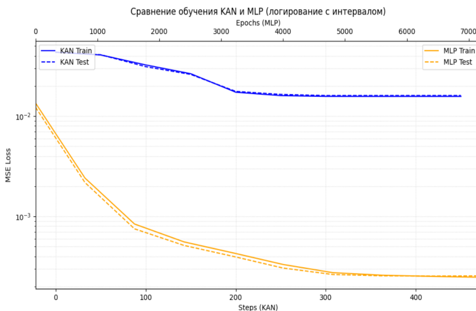
Рисунок 1 Кривые обучения KAN и MLP
