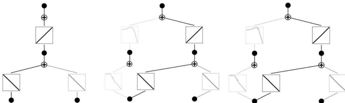
Рисунок 3 Визуализация архитектуры KAN при разных уровнях шума (0%, 3%, 7%)
