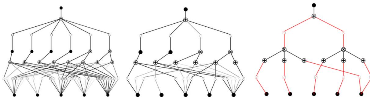
Рисунок 3 Конечная конфигурация MultKAN [5,[4,2],1] и MultKAN [5,[2,2],1] и karpiler
